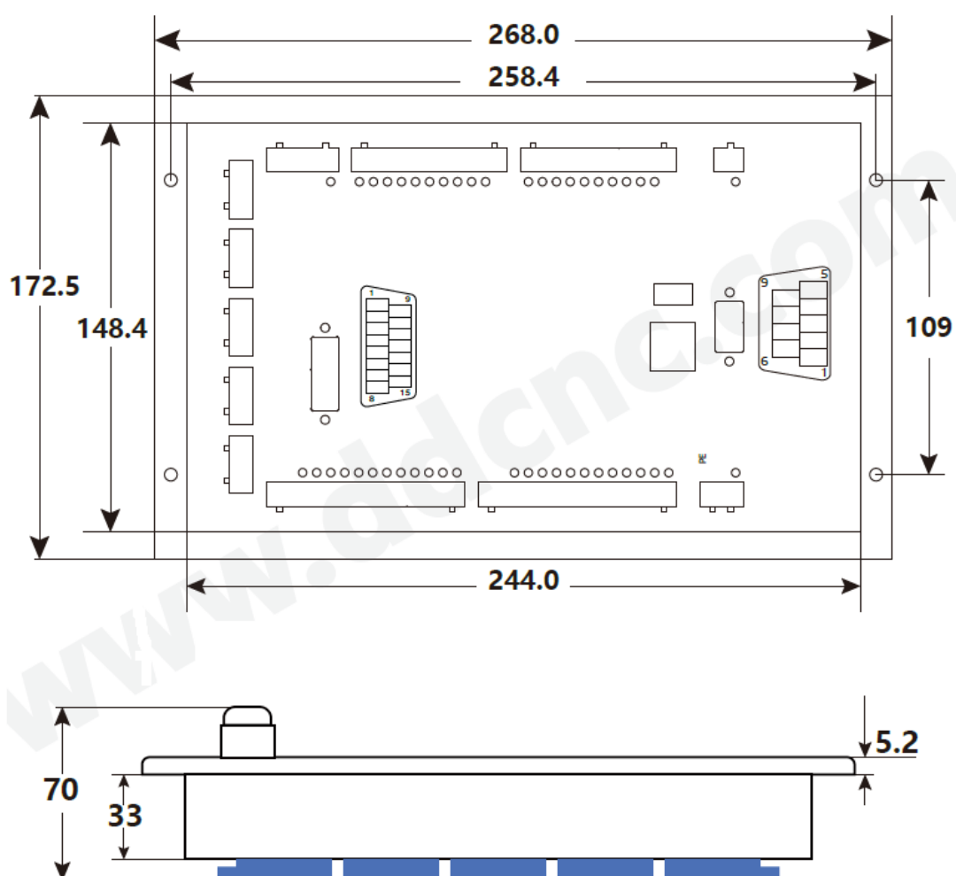
Рисунок 1 – Габаритные размеры. [Есть вектор стр.6]
