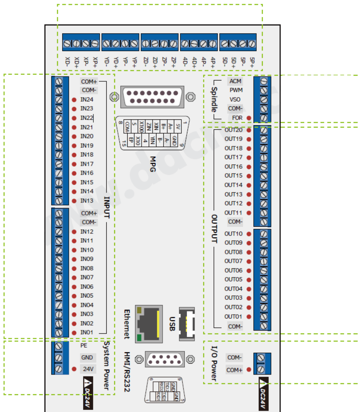
Рисунок 5 – Порты контроллера. [Есть вектор стр.16]
