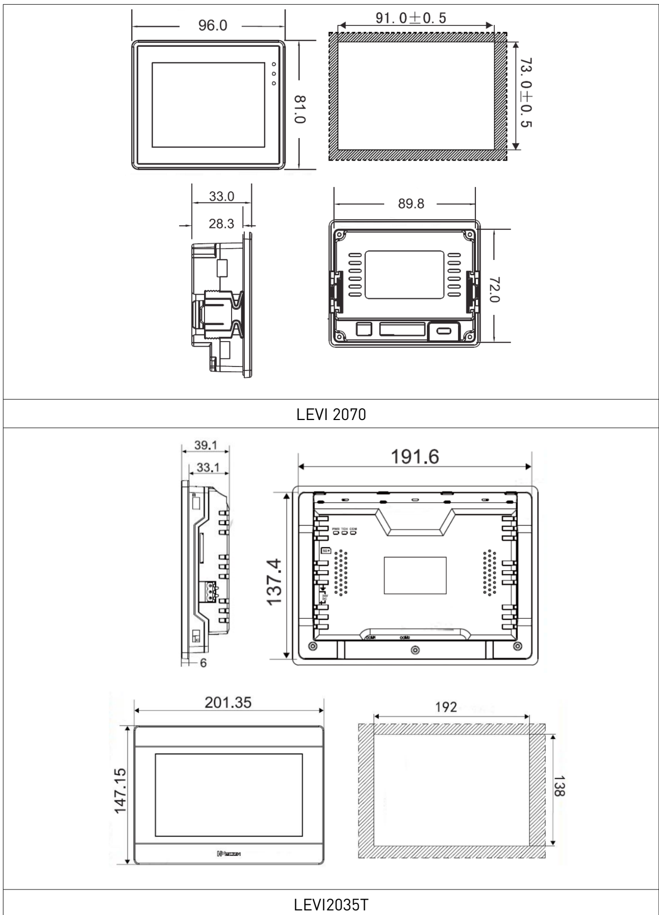
Рис. 2. Габаритные и установочные размеры модуля HMI
