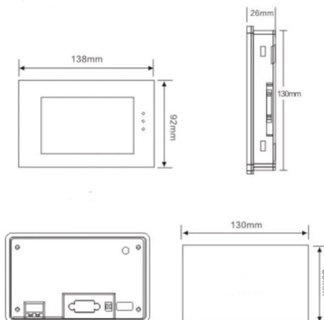
Рис. 1. Габаритные и установочные размеры модуля HMI LN043NA
