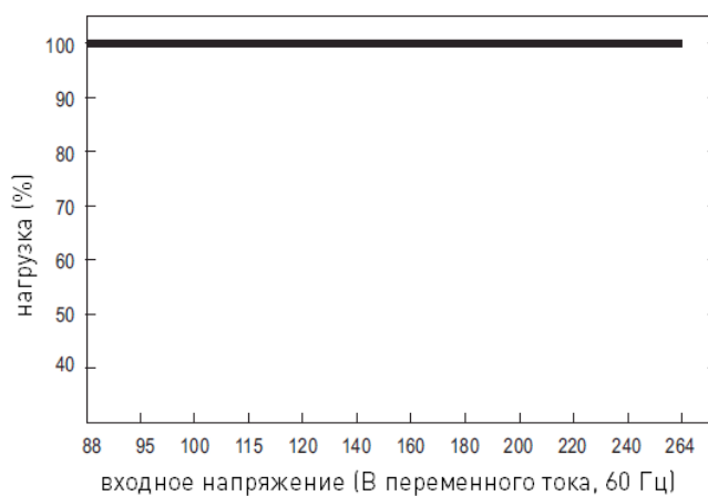
Рис. 5. Зависимость нагрузки от входного напряжения
