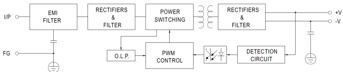
Рис. 3. Принципиальная электрическая схема
