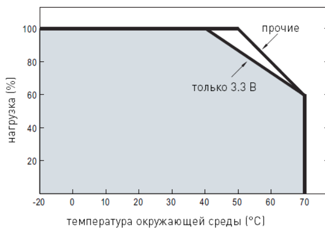
Рис. 4. Зависимость нагрузки от температуры окружающей среды
