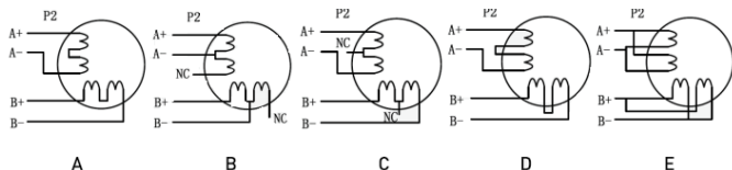
Рис. 2. Возможные схемы подключения обмоток шаговых двигателей
