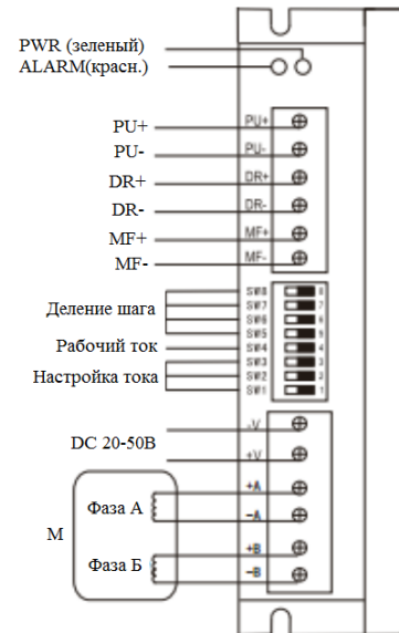
Рис. 2. Подключение драйвера
