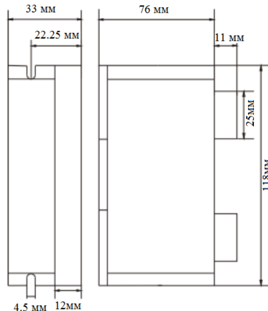
Рис. 1. Размеры устройства
