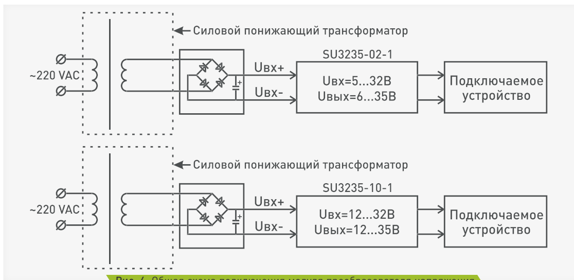
Рис. 4. Общая схема подключения модуля преобразователя напряжения
