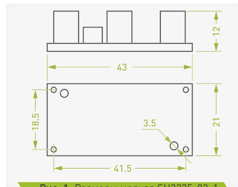
Рис. 1. Размеры модуля SU3235-02-1
