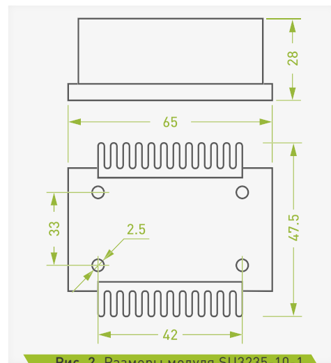
Рис. 2. Размеры модуля SU3235-10-1
