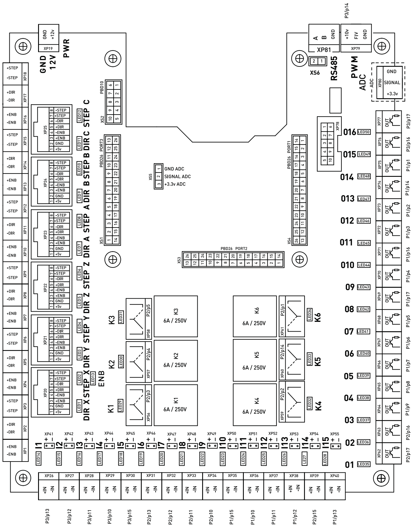
Рис. 3. Подключение модуля
