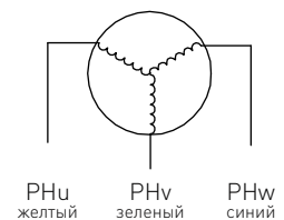
Подключение двигателя
