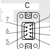
Подключение энкодера
