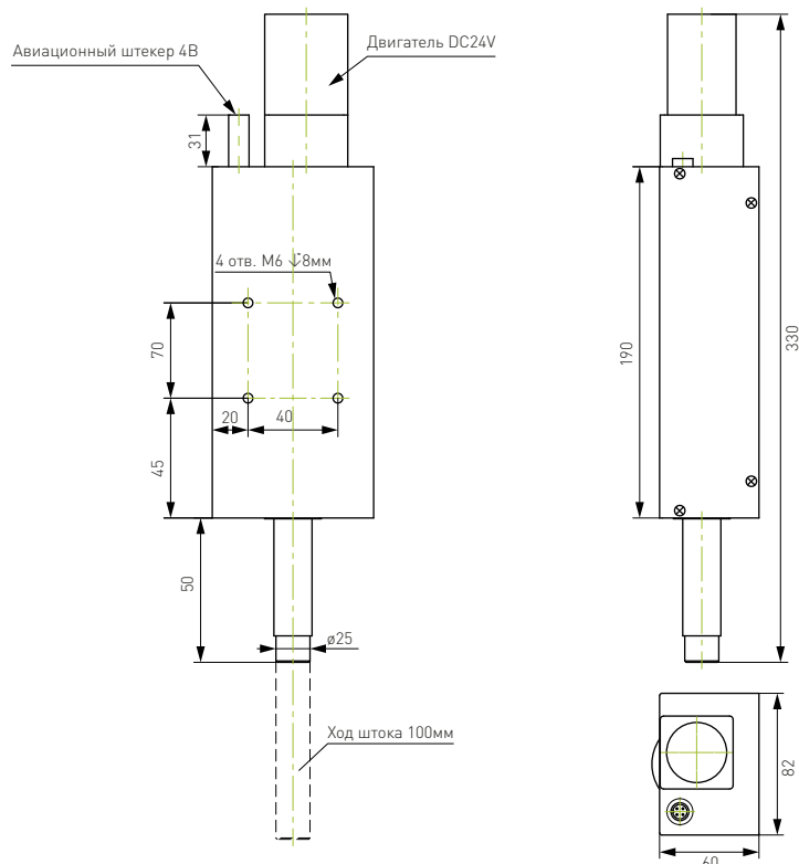
Рисунок 1 – Габаритные и присоединительные размеры подъемника резака ACM100.
