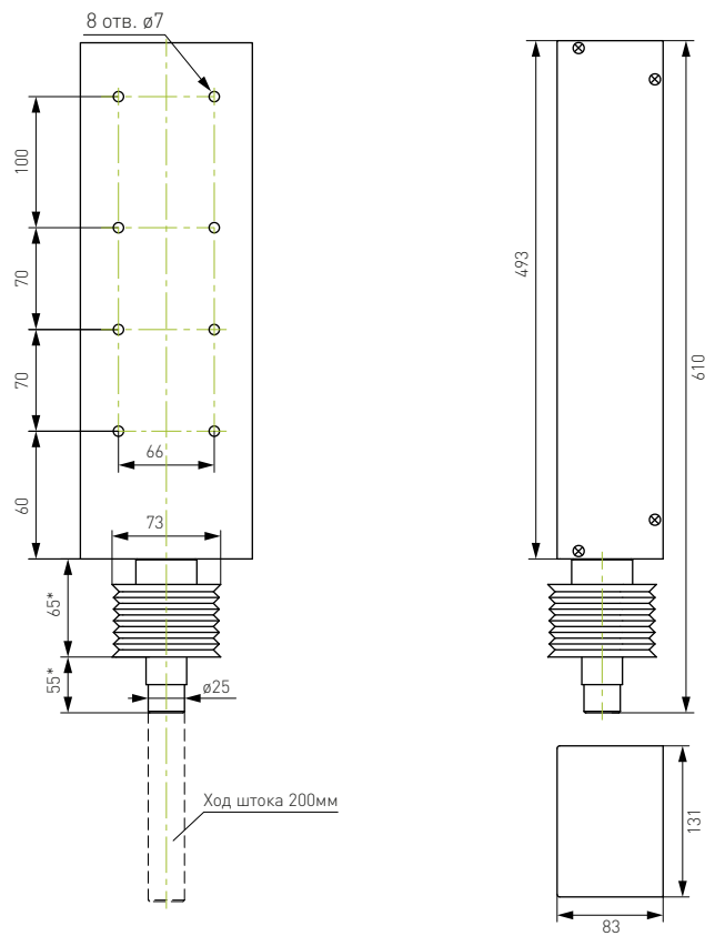
Рисунок 4 – Габаритные и присоединительные размеры подъемника резака ACM200.
