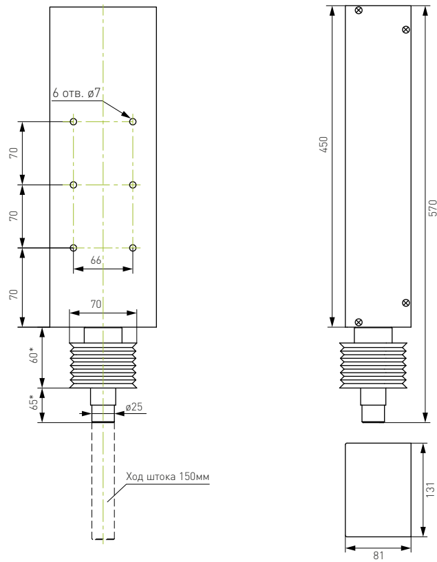
Рисунок 3 – Габаритные и присоединительные размеры подъемника резака ACM150.
