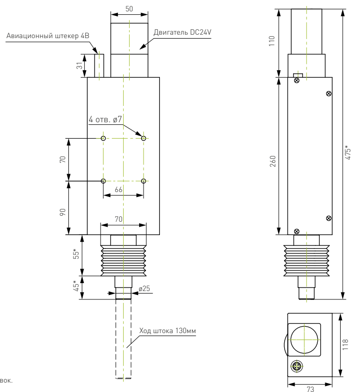
Рисунок 2 – Габаритные и присоединительные размеры подъемника резака ACM130.
