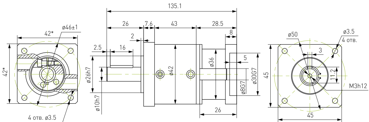
Рис. 3. Габаритные и установочные размеры редуктора планетарного 42PLF20K-8S-D10
